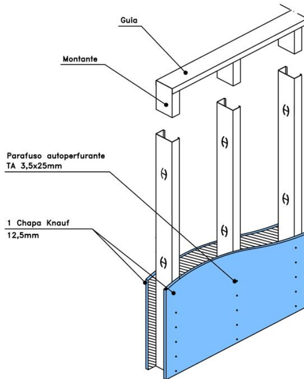
Figura 5 – Esquema de montagem parede drywall.
